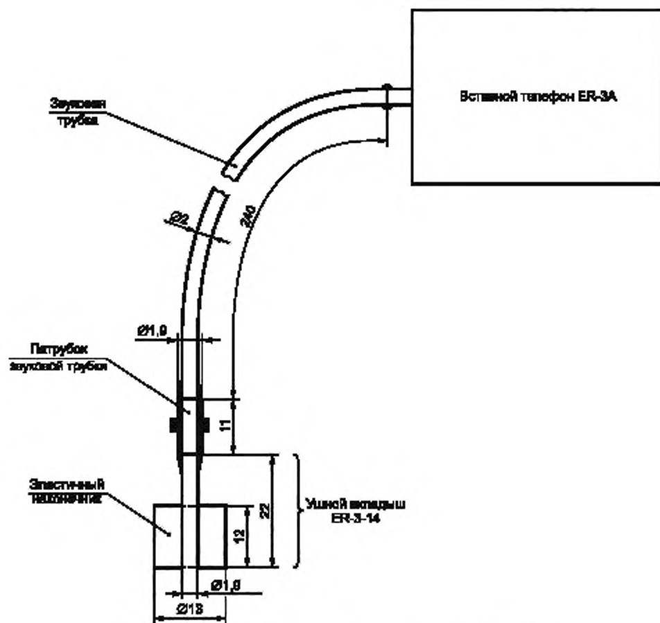
Рисунок 1 — Вставной телефон ER-3A и ушной вкладыш ER-3-14
