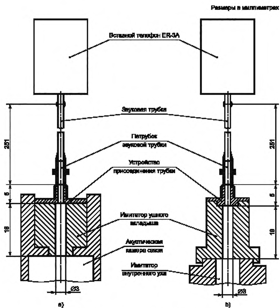
Рисунок 2 — Присоединение вставного телефона
