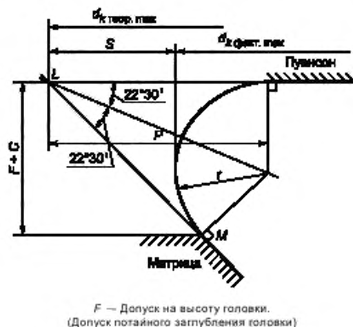
Рисунок А.1 — Схема формирования внешнего контура головки
