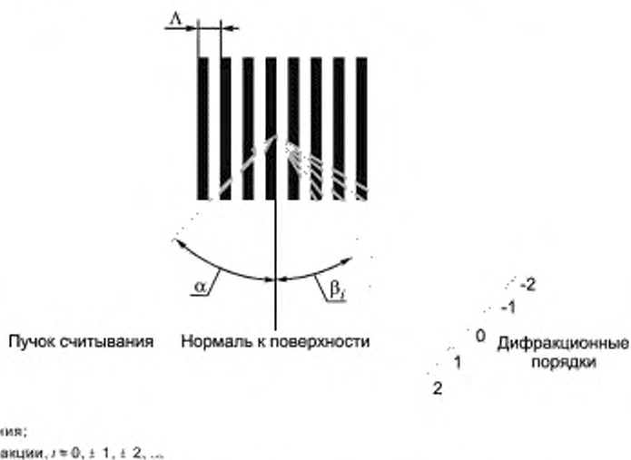
Рисунок А.2 — Дифракция пучка считывания на дифракционной решетке
