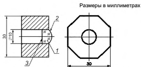
1 — эталонная линза; 2 — тороидальная поверхность; 3 — плоская поверхность
