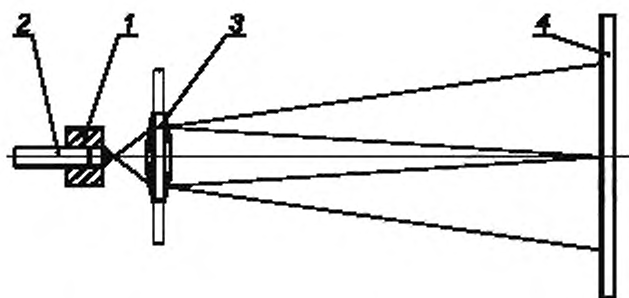
Рисунок А.2 — Схема проверки правильности установки эталонной линзы в восьмигранной оправе
