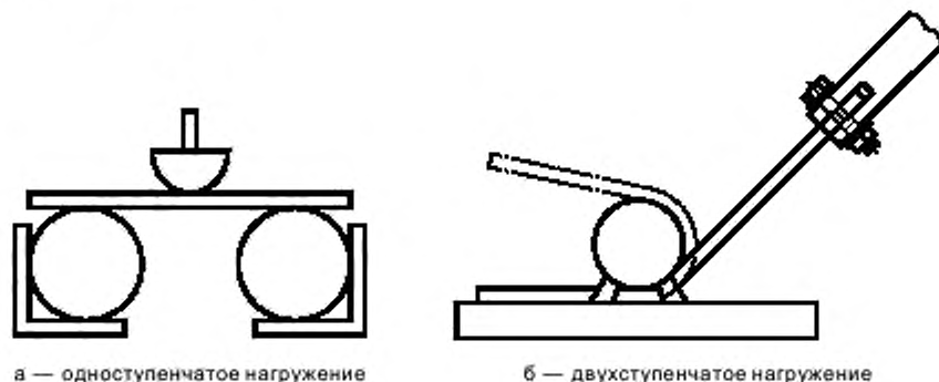
Рисунок 2 — Методы нагружения для придания образцам U-образной формы
