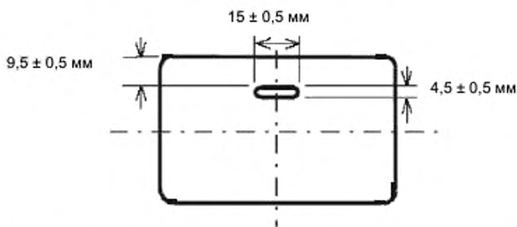
Рисунок В.2 — Щелевое отверстие, расположенное вдоль широкой кромки карты
