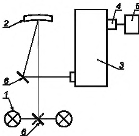
Рисунок 1 — Блок-схема установки для измерения СПЭО
