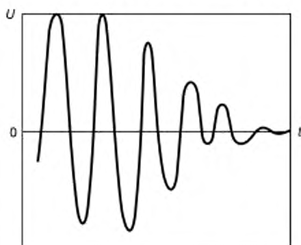
а) неповрежденная катушка
