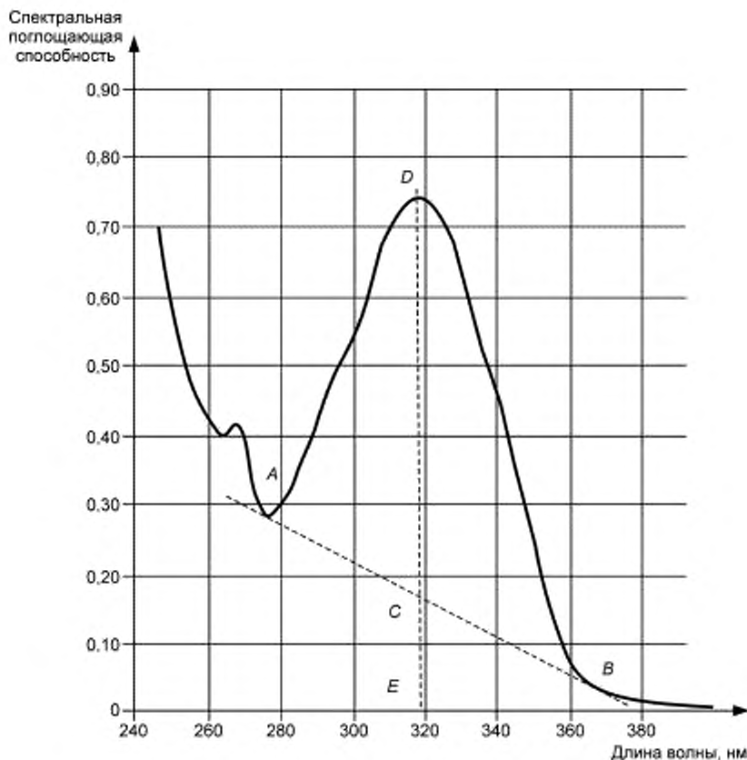
Рисунок 1 — Типичная кривая спектральной поглощающей способности
