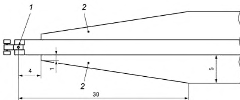
1 — точка расположения глаз оператора; 2 — заднее боковое поле обзора
