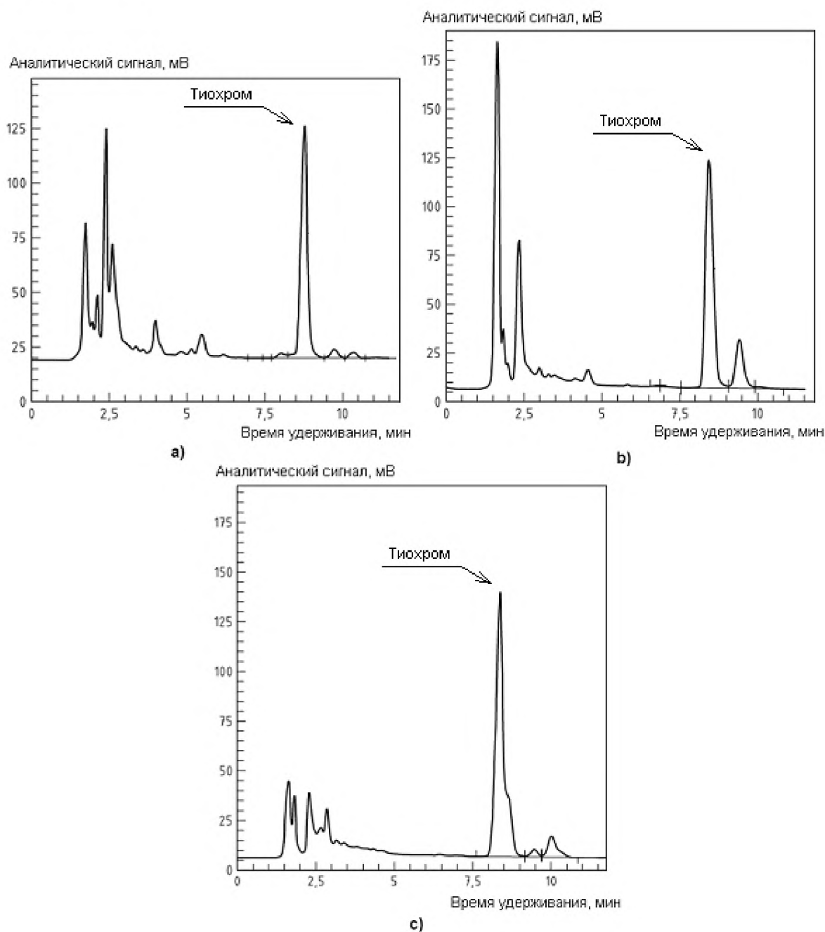
Рисунок В.2 — Примеры хроматограмм экстрактов проб салата (а), вареного риса (b) и вареной свинины (с) с добавлением градуировочного раствора тиамин с применением послеколонной дериватизации
