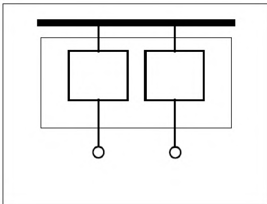
Вид внутреннего разделения 2a: выводы не отделены от сборных шин
