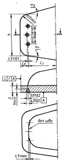
Рисунок 1 – Передняя часть Ботинка формы N (северная)
