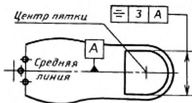
Рисунок 3 – Положение центра пятки
