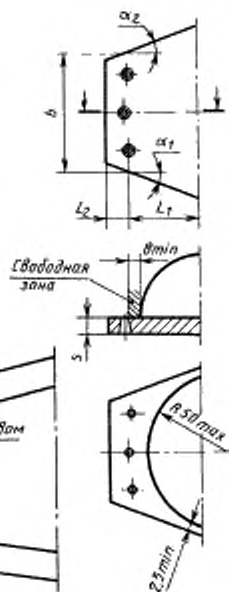
Рисунок 2 – Передняя часть ботинка форм R (гоночная) и T (туристская)
