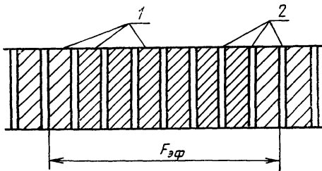
1—изображение промежутков между пластинами коллиматора на снимке; 2—изображение пластины коллиматора на снимке; F_{эф} —размер фокусного пятна, мм
